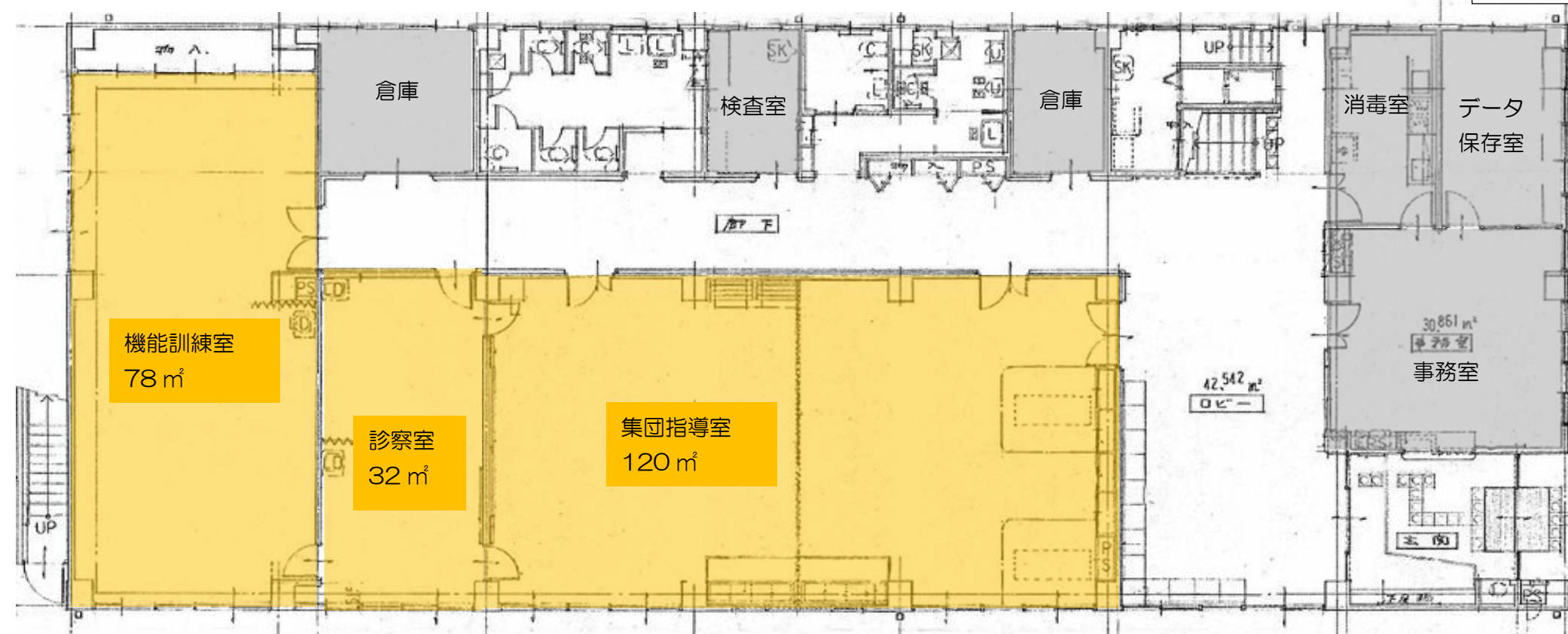
1 階平面図
