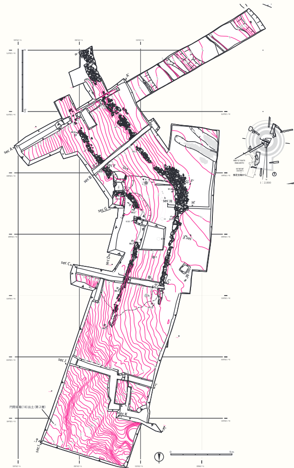
第 60 図 クレビレ部東側遺構平面図 1 : 150
